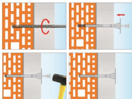
povrchová montáž
